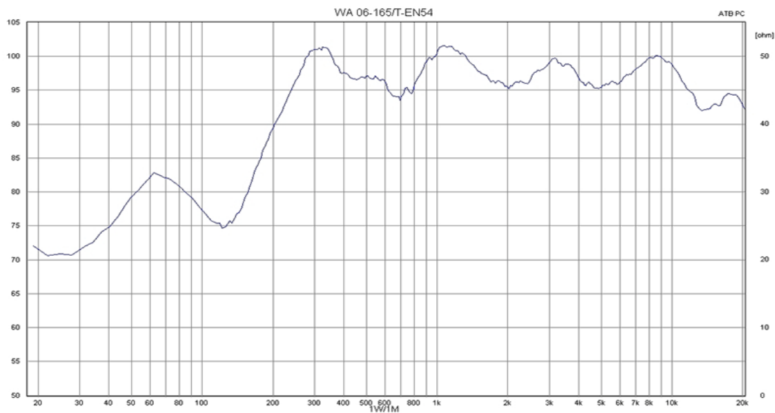
Diagramma della risposta in frequenza
