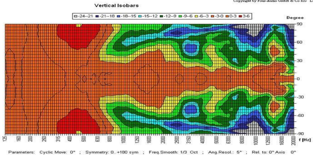
Diagramma della risposta in frequenza
